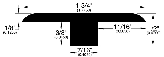
T-Mold (295)
