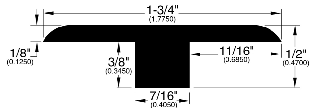
T-Mold (295)
