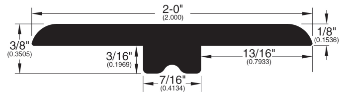
T-Mold (289)
