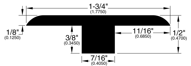
T-Mold (295)
