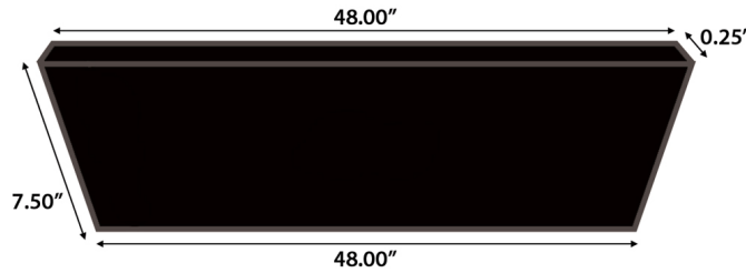
48" Riser
